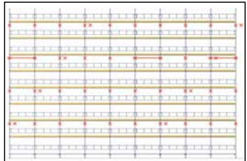
Stagning med skyddsräcksram GFL/GFLH och förankring
