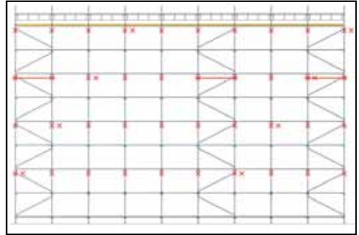
Stagning med vertikala diagonalstag och förankring
